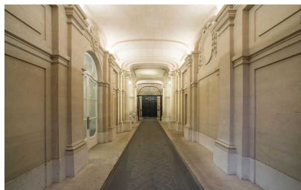
17.60 mètres (8x70cm + 8x1.5cm) de linéaire 5655-Lignon à 120 LED de puissance en blanc chaud, optique 120°, éclairent les voûtes du porche.
